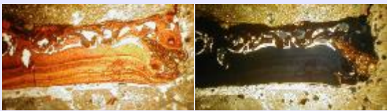
Vidrio producido por choque con una textura de flujo y algunos fragmentos minerales procedente de la estructura de impacto de Azuara (brecha polimítica sita cerca de Sta. Cruz de Nogueras). El vidrio puede observarse al microscopio bajoluz paralela (izquierda) y nicoles cruzados (derecha).
