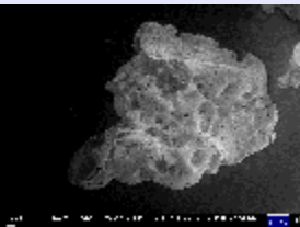
Izquierda: Carbón amorfo, probable vidrio de carbón procedente del fundido por choque de carbonos de la Fm. Utrillas. Muestra procedente de la cuenca de impacto de Rubielos de la Cerdá (cerca de Cutanda- Barrachina). Derecha: Fluidización enigmática de nódulos de chert presentes en calizas del Jurásico. Muestra, cortesía de Daniel Gorgas, procedente de la estructura de impacto de Azuara (al sur de Fuendetodos).
