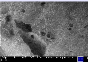
Probable roca de fundido de sulfato cálcico (yeso/anhidrita). Derecha: la roca vesicular bajo el microscopio electrónico de barrido. Muestra procedente de la cuenca de impacto de Rubielos de la Cerdá (cerca de Cutanda- Barrachina).
