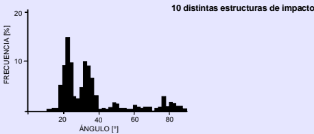
Histograma de la orientación de PDFs generadas por impacto. 351 conjuntos de PDFs provenientes de 10 estructuras de impacto. Según French (1999).
