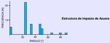
Rasgos de deformación planar en cristales de cuarzo provenientes de la estructura de impacto de Azuara. Análisis realizado por la Dra. Ann Thierault, del Geological Survey of Canada. 48 conjuntos.
