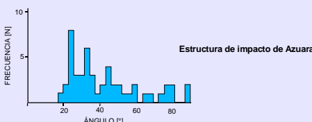
Rasgos de deformación planar en cristales de cuarzo provenientes de rocas de la estructura de Azuara. Análisis efectuados por Eugenio Guerrero Serrano, de la universidad Complutense de Madrid. 90 conjuntos.
