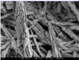
Cristalitos de fundido de carbonato vistos bajo el microscopio electrónico de barrido. Muestra procedente de la cuenca de impacto de Rubielos de la Cerdá.
